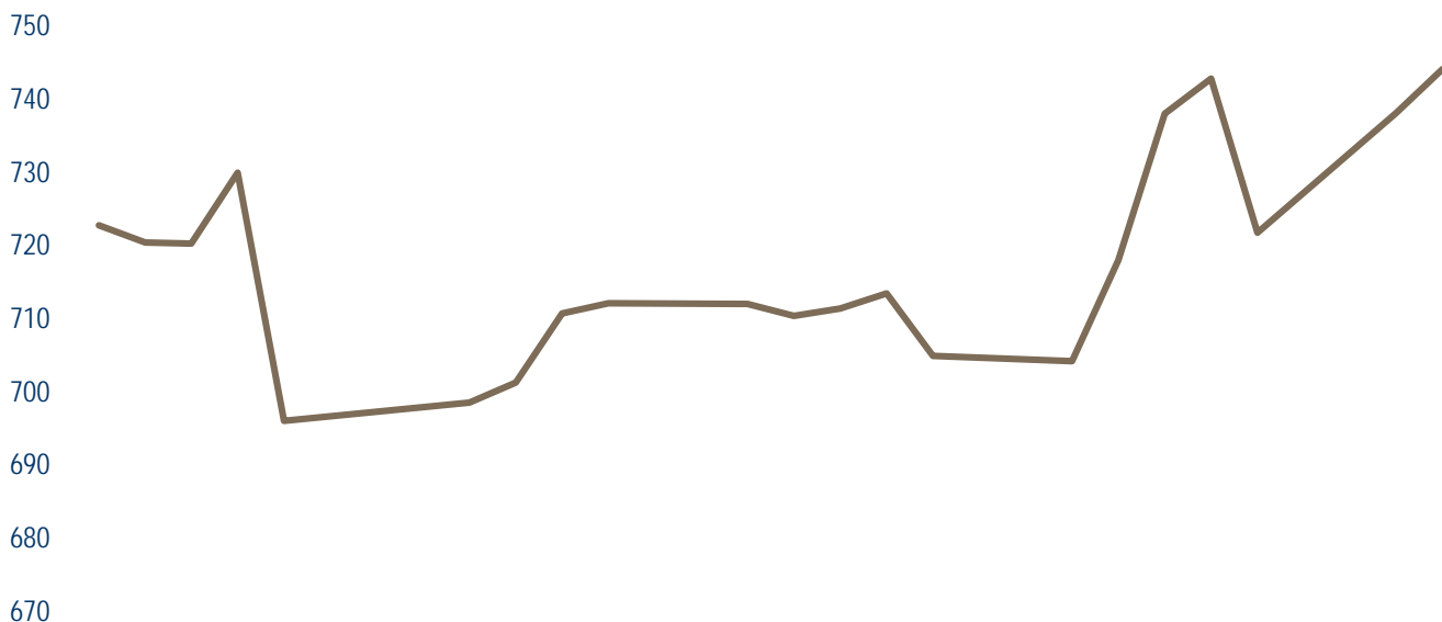
График индекса UCI за декабрь 2025 года
